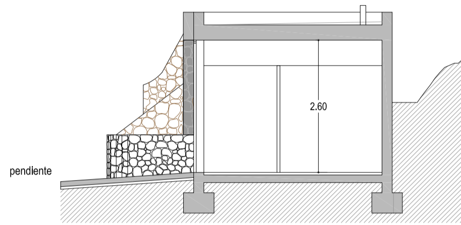
Sección A - A
